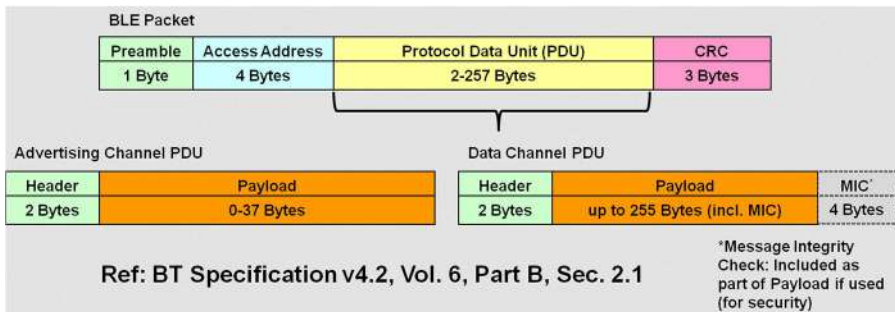
Figure 7-6. BLE packet types
